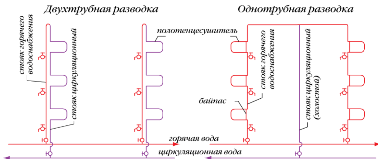
Рис. 1.1 - Схема разводки горячего водоснабжения в централизованных системах
