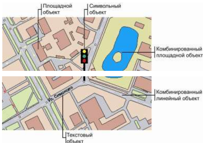
Рисунок 9.5. Примеры объектов
